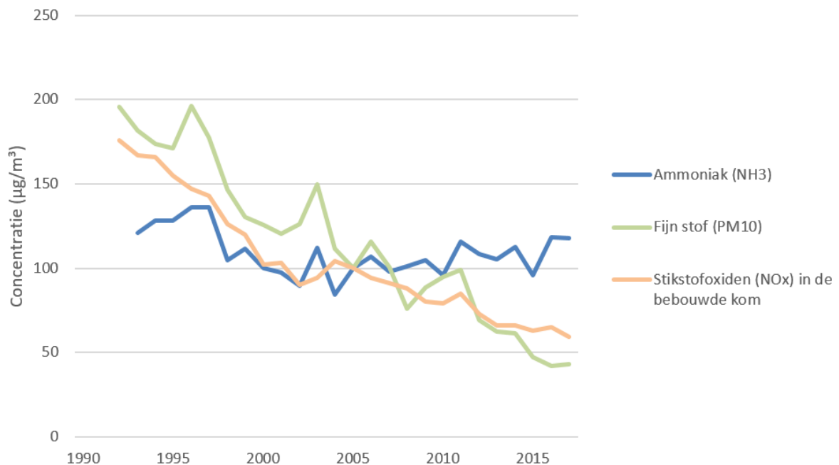
Figuur 6. Ontwikkeling concentraties ammoniak, fijn stof ( \text{PM}_{10} ) en \text{NO}_x ( \text{NO}_x : concentraties in de bebouwde kom) 1990-2017 14
